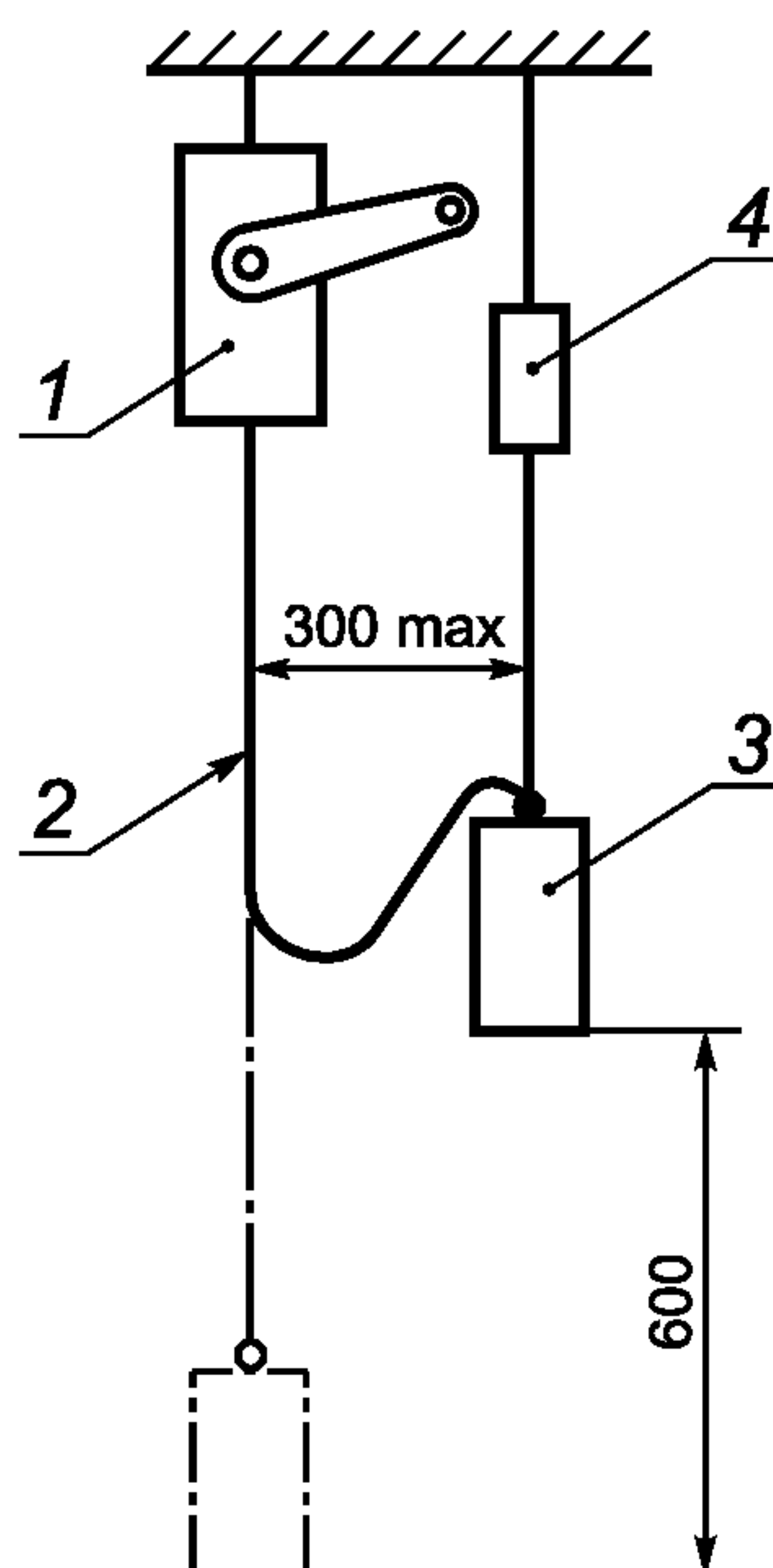
1 — спасательное подъемное устройство; 2 — строп; 3 — испытательная масса; 4 — устройство быстрого расцепления
