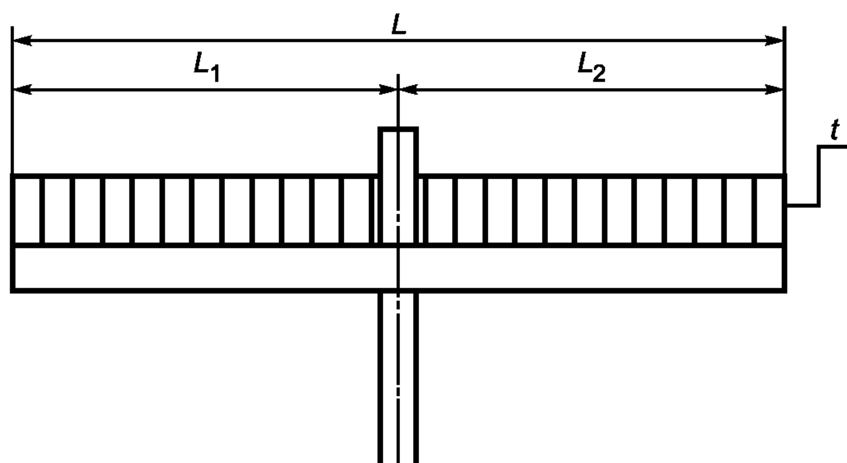
Рисунок 4 — Внецентренная нагрузка перпендикулярно центральной оси
