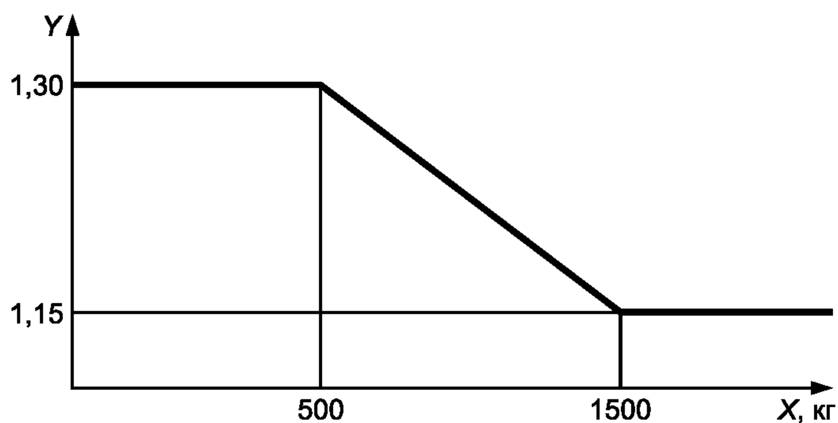
Рисунок 8 — Коэффициент f как функция номинальной нагрузки
