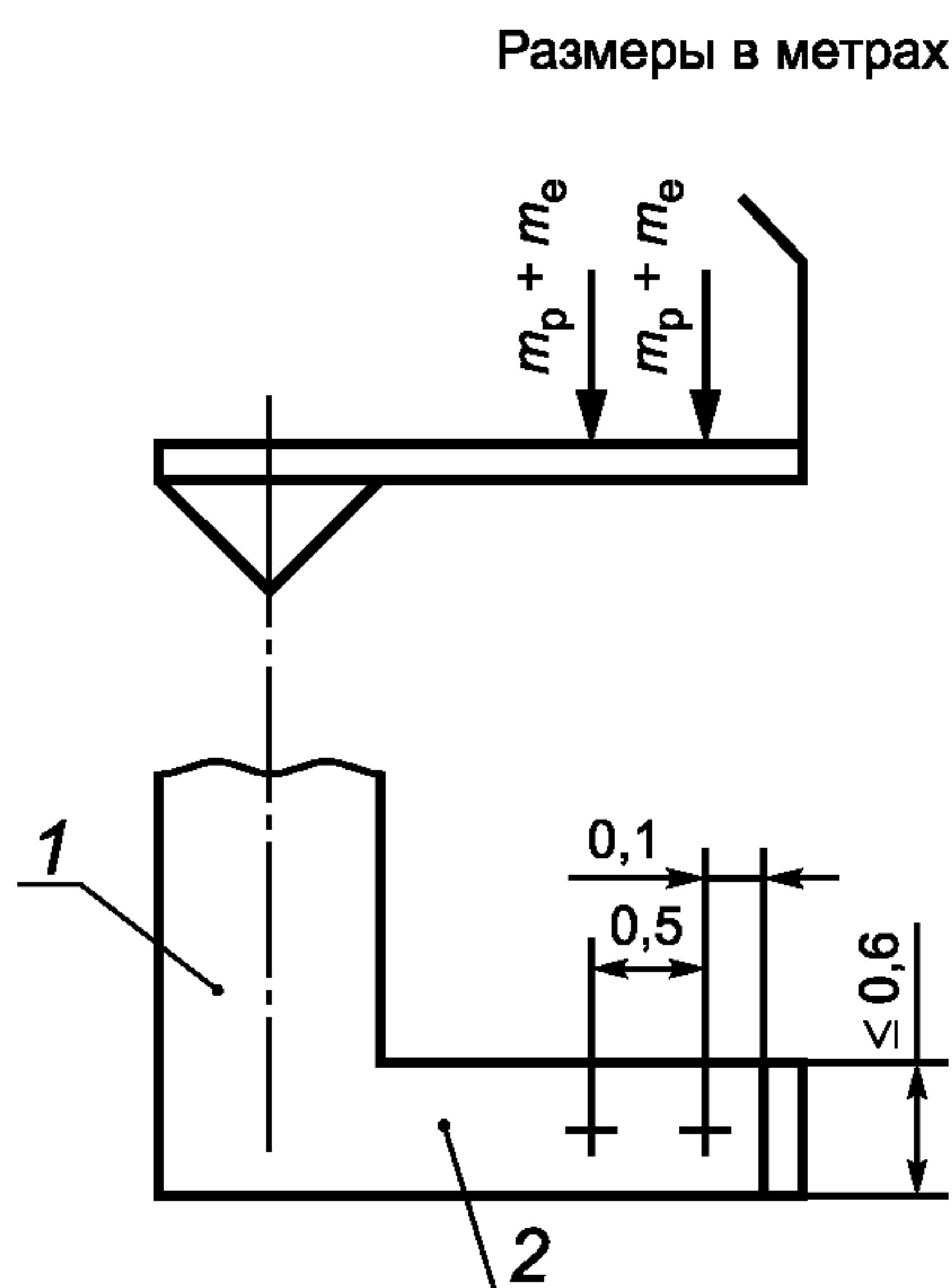
1 — основная рабочая платформа; 2 — расширитель рабочей платформы
