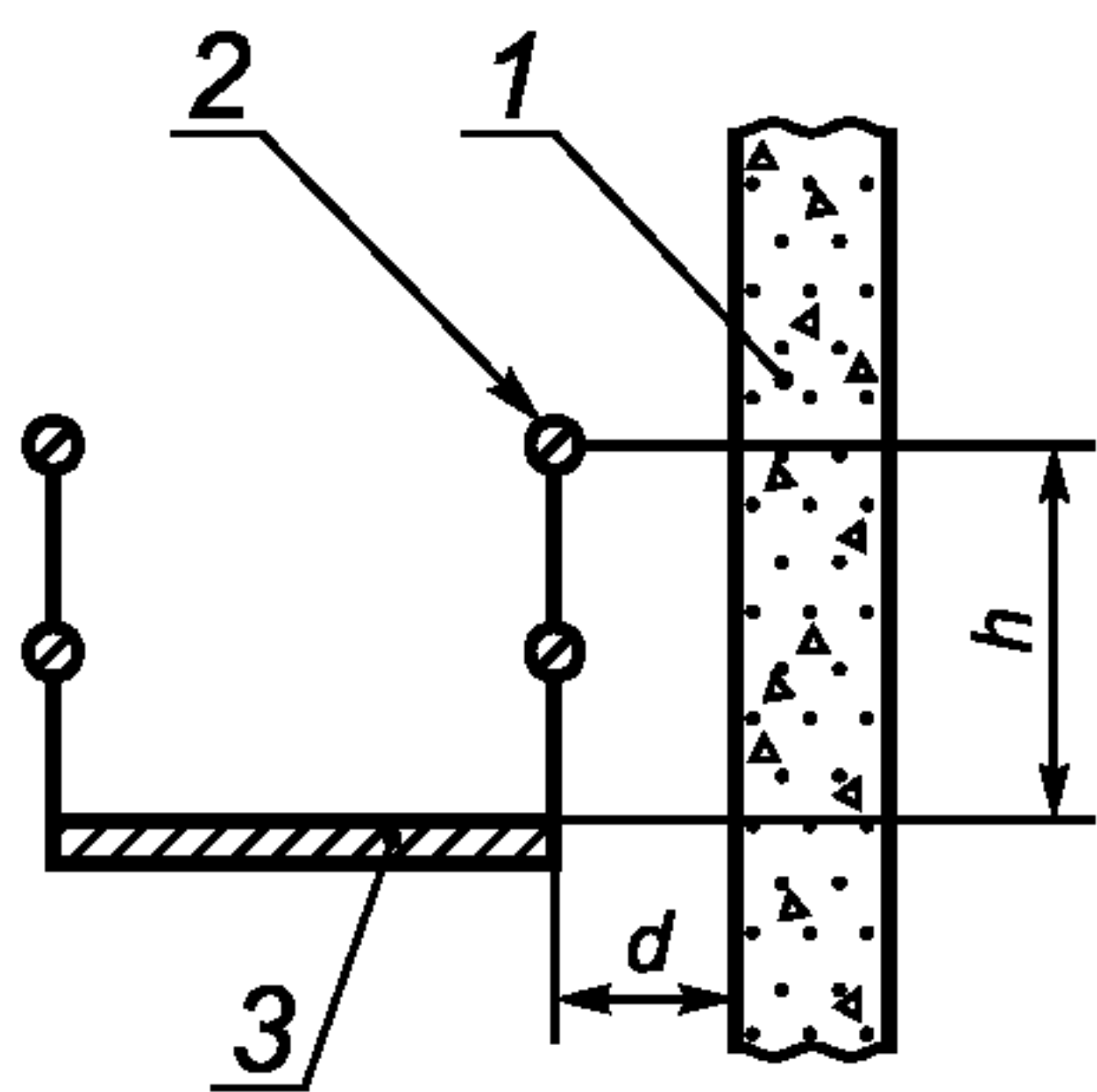
1 — стена; 2 — поручень; 3 — рабочая платформа
