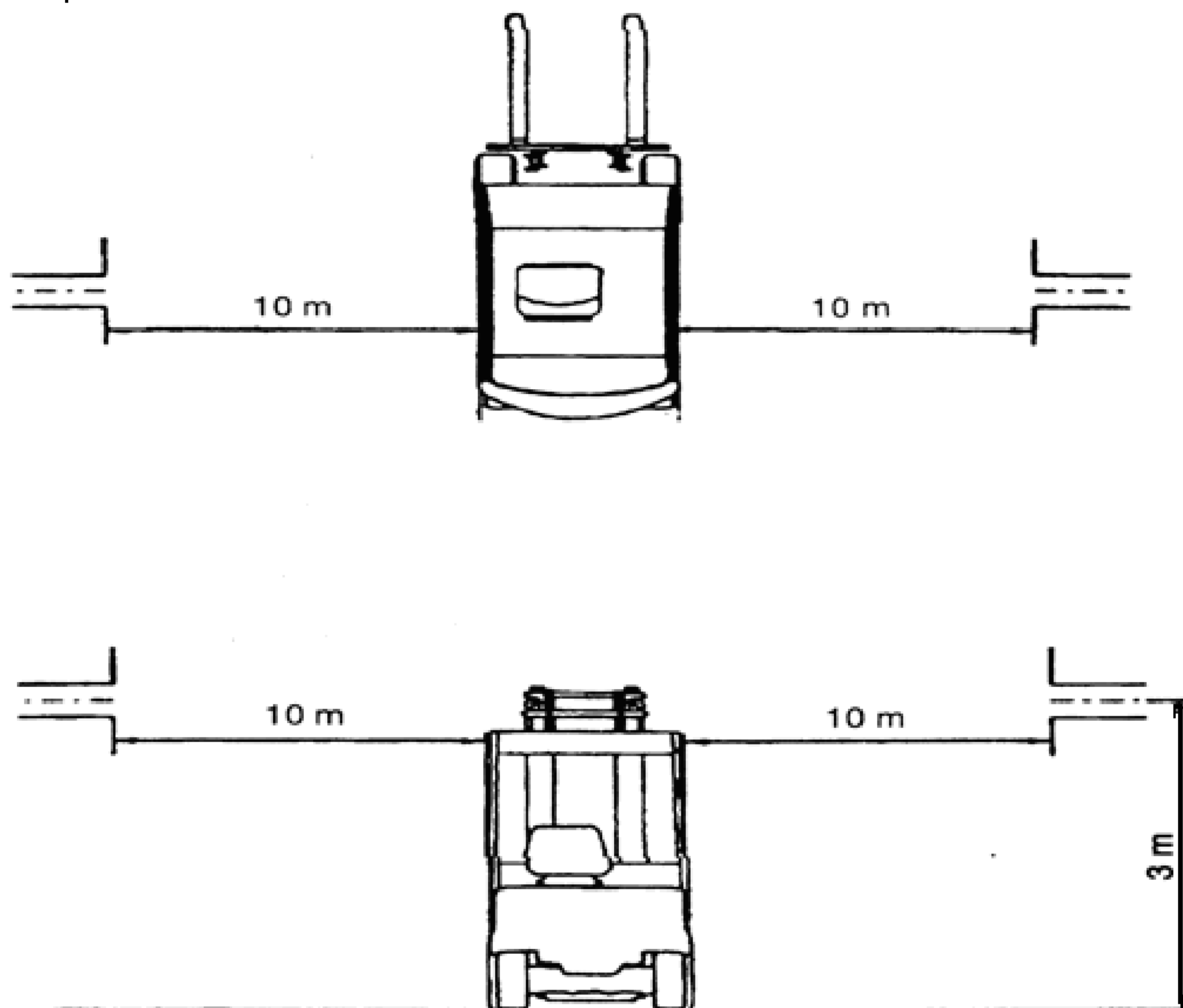
Рисунок 2 – Испытание на помехоэмиссию
