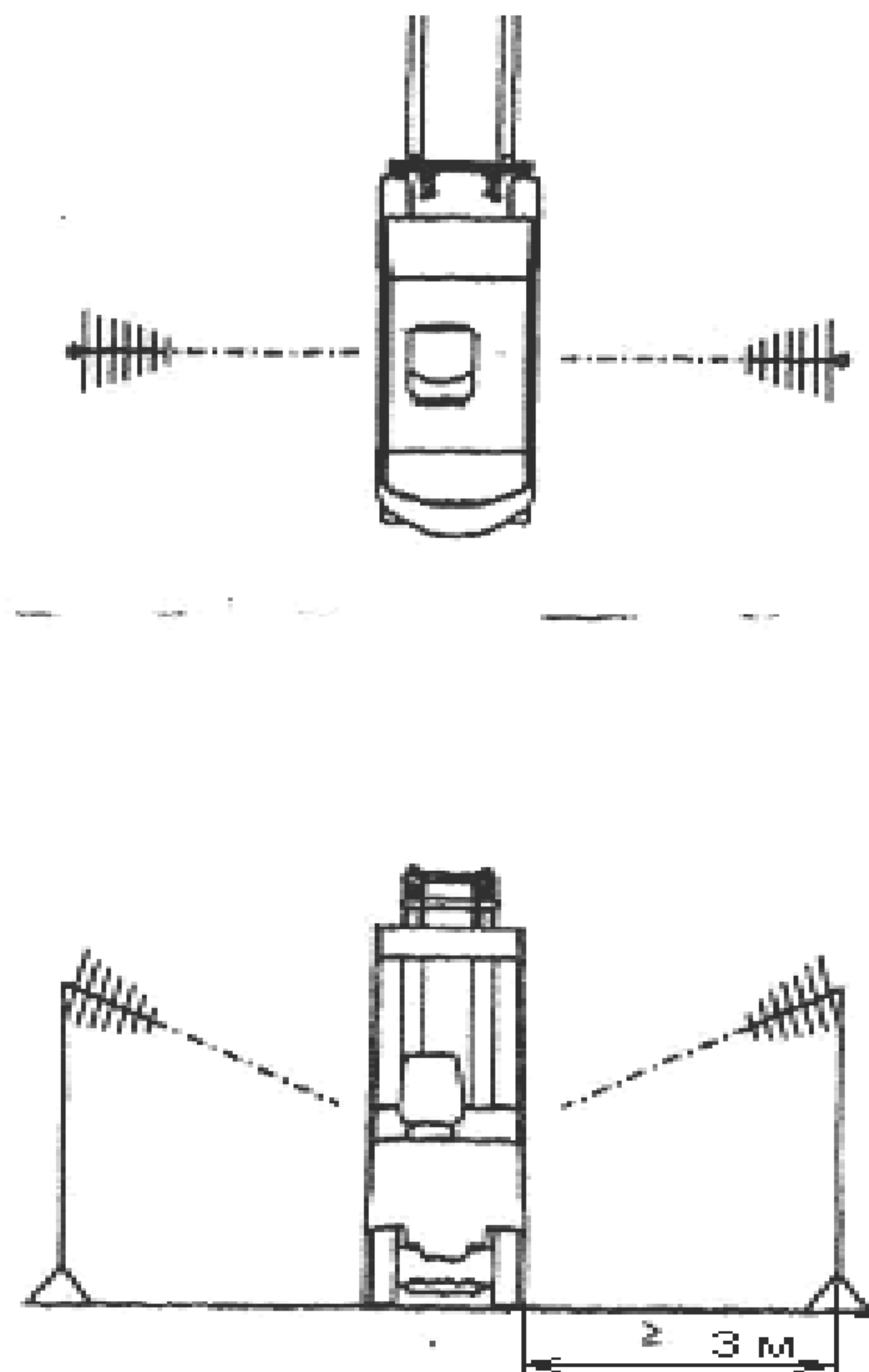
Рисунок 3 – Испытание на помехоустойчивость
