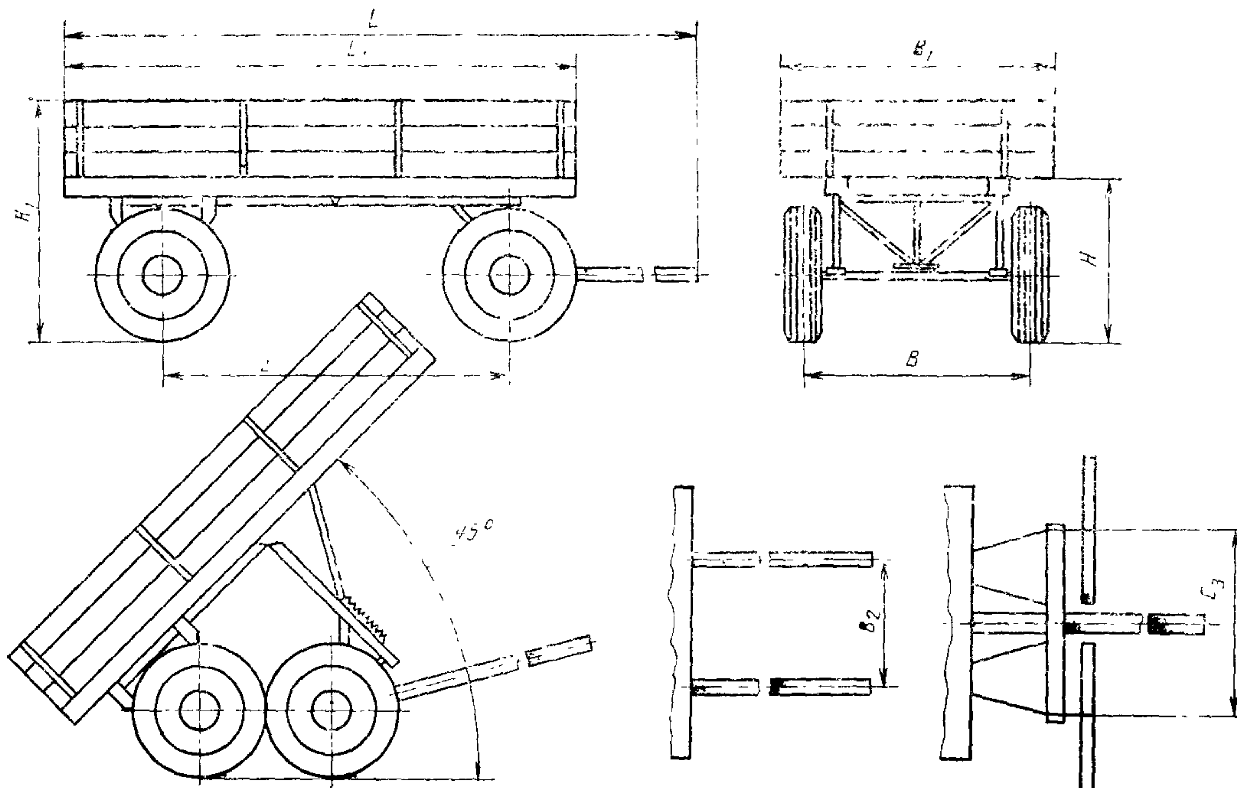
Вид повозки с наклонным кузовом
